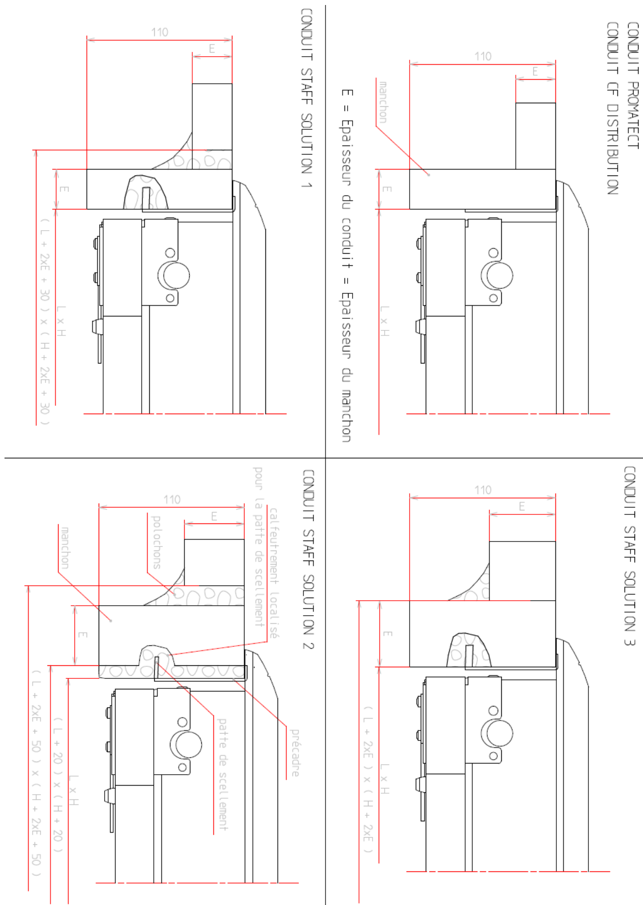
Figure 6 : Type de montage sur conduit
