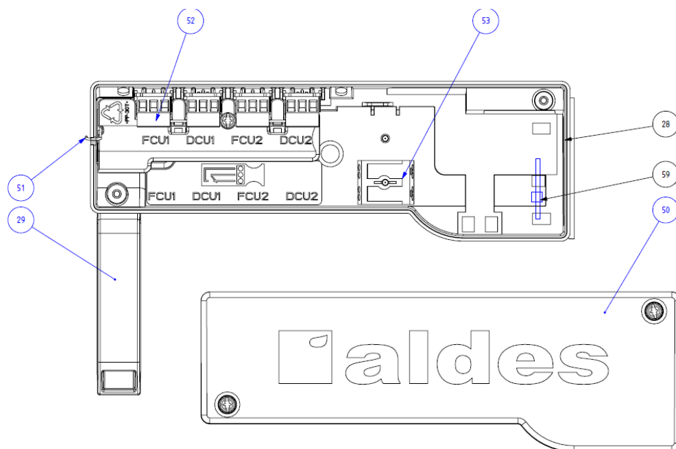
VUE SOUS ENSEMBLE BOITIER PRINCIPAL PL-1207 indice A
