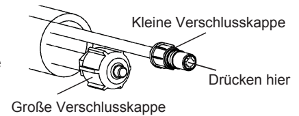
Große Verschlusskappe
