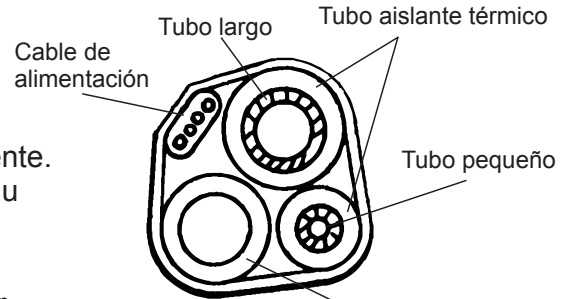
Manguera de drenaje (preparado por el usuario)
