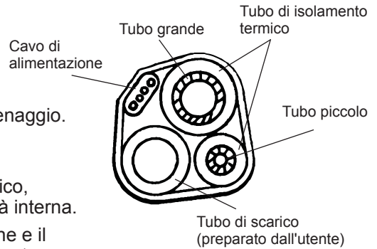
Isolamento termico
