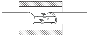
Wärmedämmung
