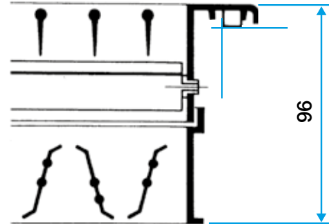
Grille AC 102 D avec registre AGB ou SGS monté
