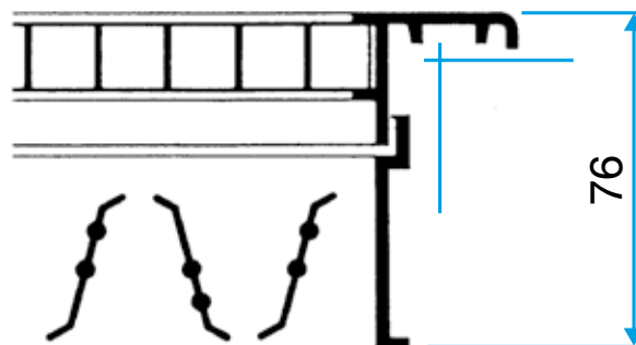
Grille AC 123 avec registre AGB ou SGS monté
