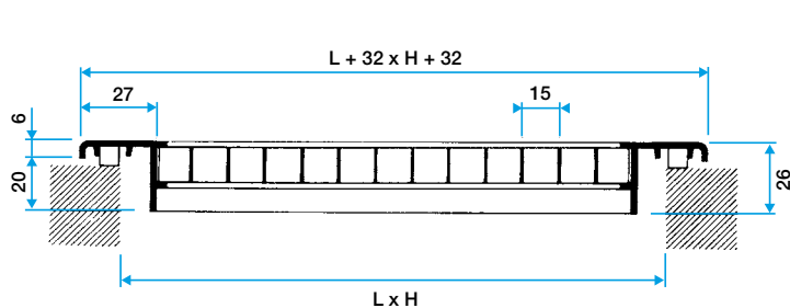
Grille AC 123 seule
