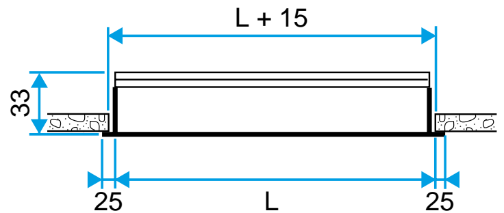
Diffuseur ALD 610 - 620
