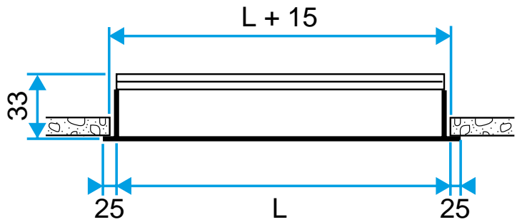
Diffuseur ALD 610 - 620
