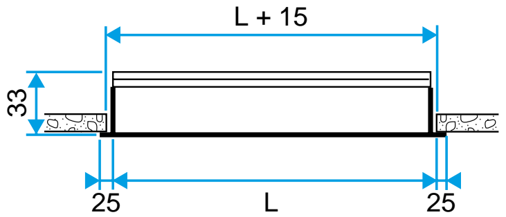
Diffuseur ALD 610 - 620
