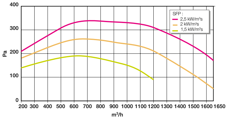
Caractéristiques aérauliques et consommation d'énergie DFE COMPACT 1600
