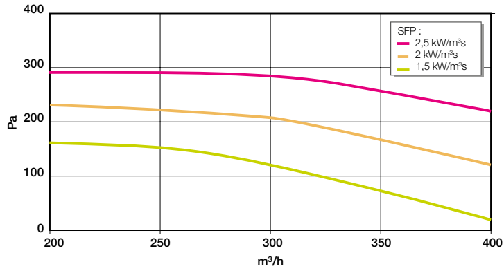
Caractéristiques aérauliques et consommation d'énergie DFE COMPACT 450
