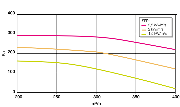
Caractéristiques aérauliques et consommation d'énergie DFE COMPACT 450
