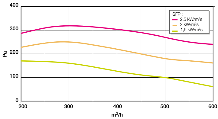
Caractéristiques aérauliques et consommation d'énergie DFE COMPACT 600
