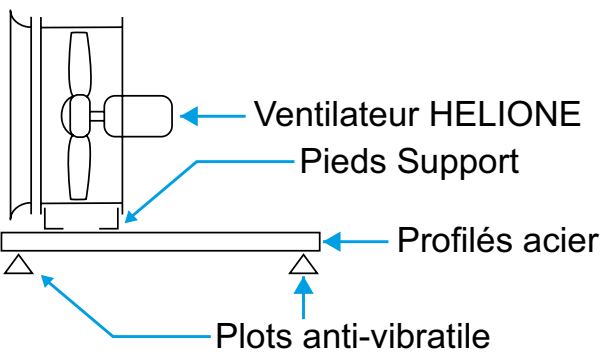
Montage sur structure avec HELIONE virole courte
