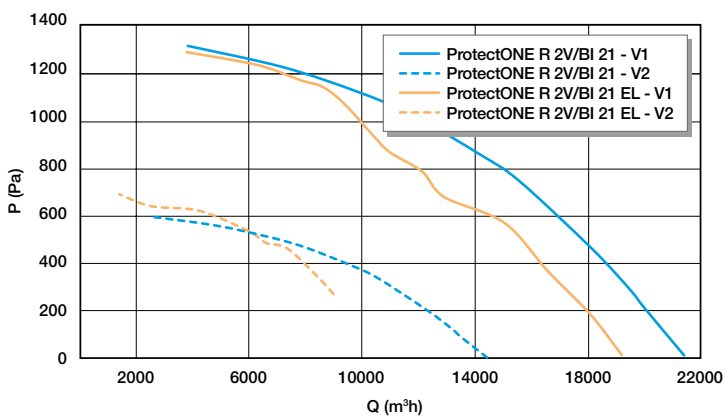
Aeraulic properties ProtectONE® R 21.0 EL - 2SP - BI
