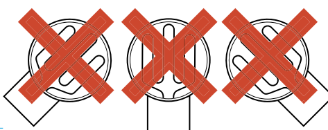
La position boîtier «tête en bas» est déconseillée pour un bon fonctionnement des limiteurs (automatique et manuel).
