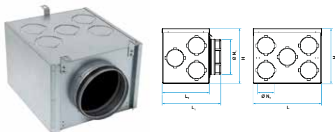
Caisson métallique OPTIFLEX 10P
