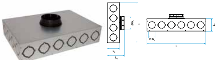
Caisson de répartition OPTIFLEX 20 piquages
