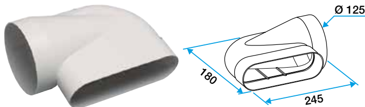
Coude 90° horizontal pour conduit
