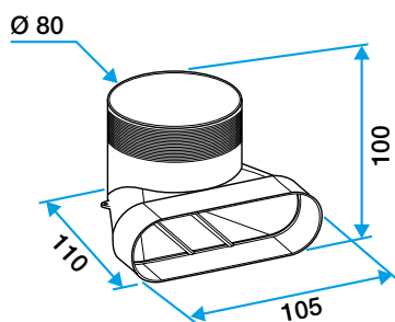
Coude mixte pour bouche Ø80 mm
