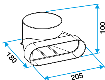
Coude 90° vertical pour bouche
