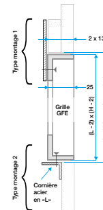
Exemple de mise en oeuvre GFE 007 - Cadre apparent
