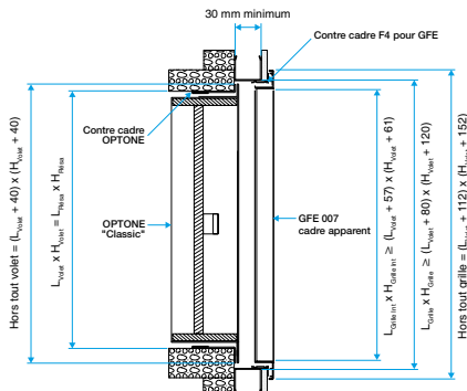
Exemple de mise en oeuvre GFE 007 - Cadre apparent
