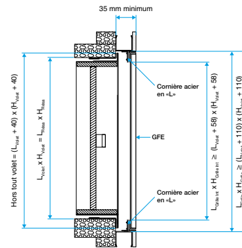
Cotes pour installation devant volet OPTONE
