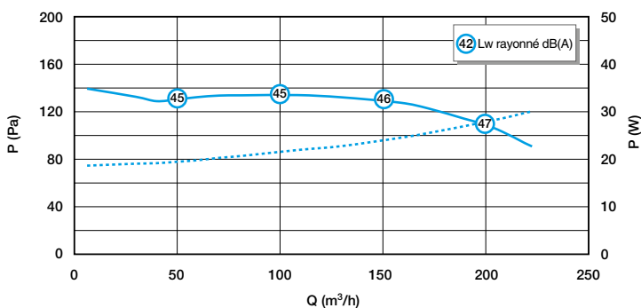
Courbe aérodynamique et acoustique EasyHOME Hygro Classic
