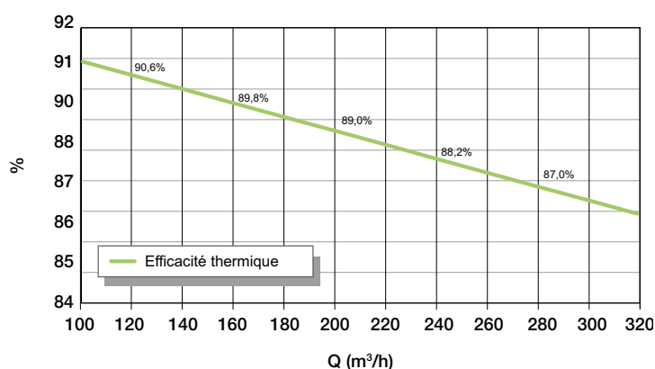
Efficacité thermique InspirAIR® Side 300 Classic DHU
