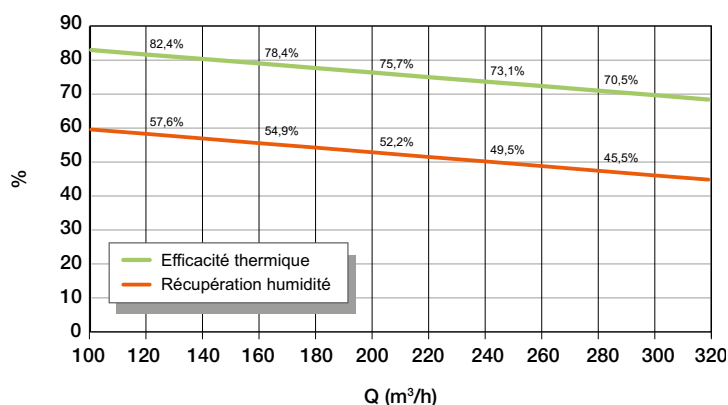
Efficacité thermique et latente InspirAIR® Side 300 Classic ERV DHU
