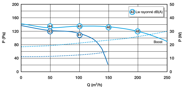
Courbe aéralique et acoustique EasyHOME Auto Classic
