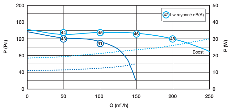
Courbe aéralique et acoustique EasyHOME Auto Classic
