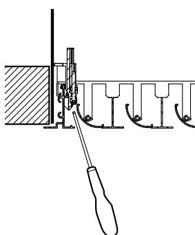
Diffuseur de soufflage avec fixation S3
