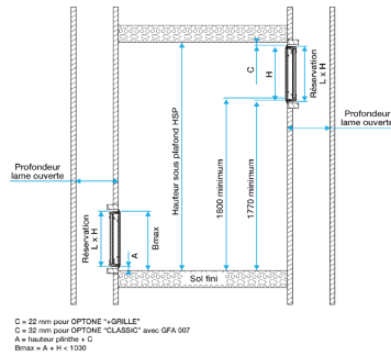
Encombrement OPTONE «Classic» 1V avec son contre-cadre (mm)
