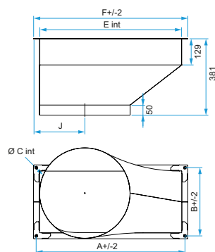
Pièce de transformation rectangulaire &gt; circulaire VEX600
