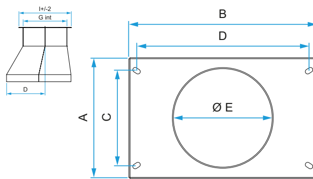
Pièce de transformation rectangulaire &gt; circulaire VEX400
