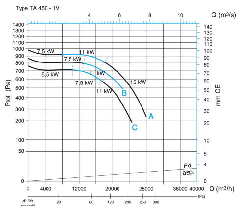
Caractéristiques aérauliques ProtectONE® TA 450 - 1V
