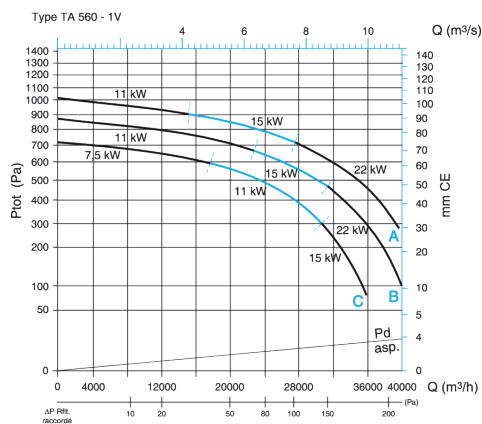
Caractéristiques aérauliques ProtectONE® TA 560 - 1V
