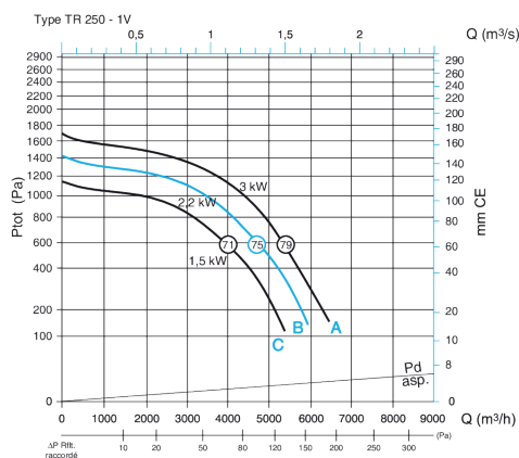
Caractéristiques aérauliques ProtectONE® TR 250 - 1V
