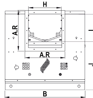
Encombrement (mm) - vue de face
