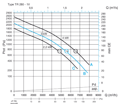
Caractéristiques aérauliques ProtectONE® TR 280 - 1V
