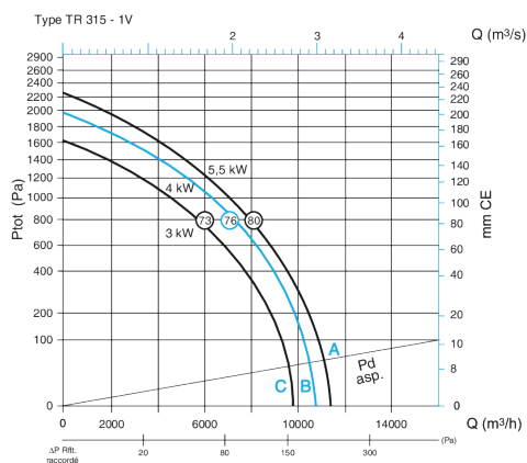
Caractéristiques aérauliques ProtectONE® TR 315 - 1V
