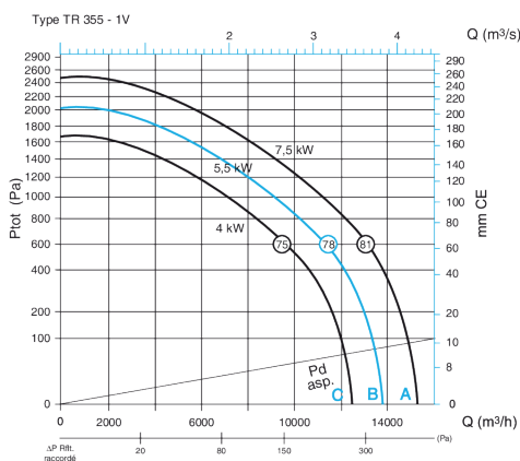
Caractéristiques aérauliques ProtectONE® TR 355 - 1V
