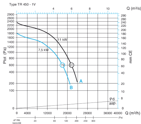
Caractéristiques aérauliques ProtectONE® TR 450 - 1V
