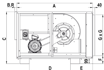
Encombrement (mm) - vue de profil
