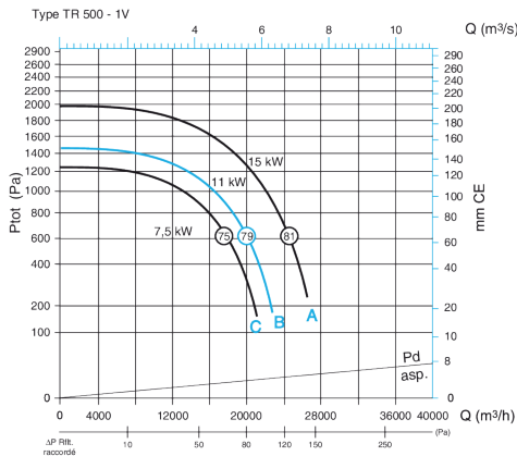
Caractéristiques aérauliques ProtectONE® TR 500 - 1V
