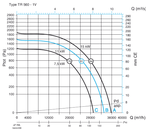
Caractéristiques aérauliques ProtectONE® TR 560 - 1V
