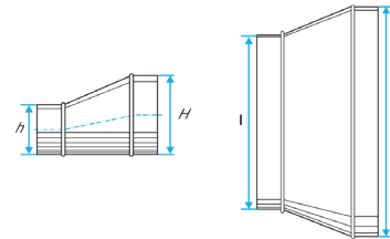
Schéma d'encombrement Réduction Oblongue Tangentielle sur Plat
