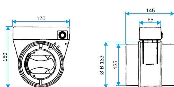
Dimensions RPM D125
