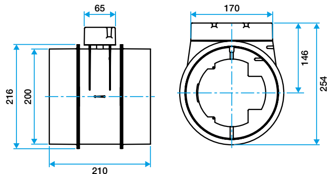
Dimensions RPM D200
