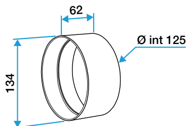
Raccord femelle Ø125 mm
