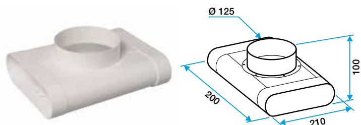
Té 90° vertical pour bouche
