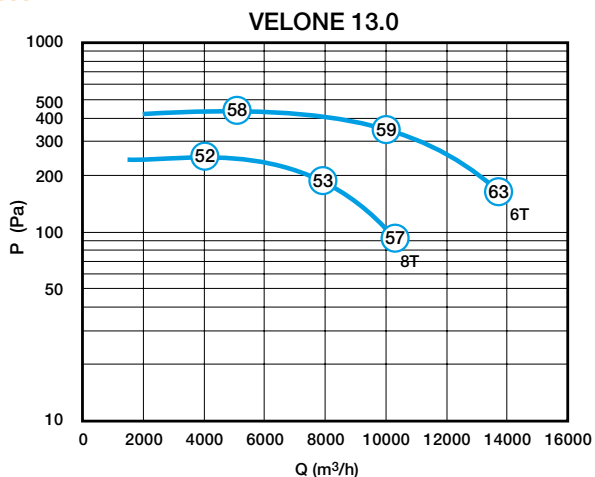
Caractéristiques aérauliques et acoustiques VELONE 13 - 6/8T 2.2/1.3 KW
