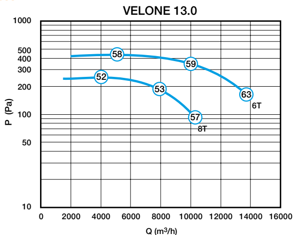
Caractéristiques aérauliques et acoustiques VELONE 13 - 6T 2,2 KW
