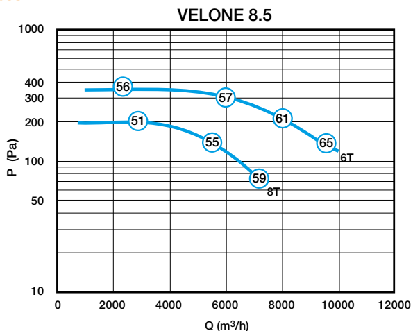
Caractéristiques aérauliques et acoustiques VELONE 8.5 - 6T 1.1KW
