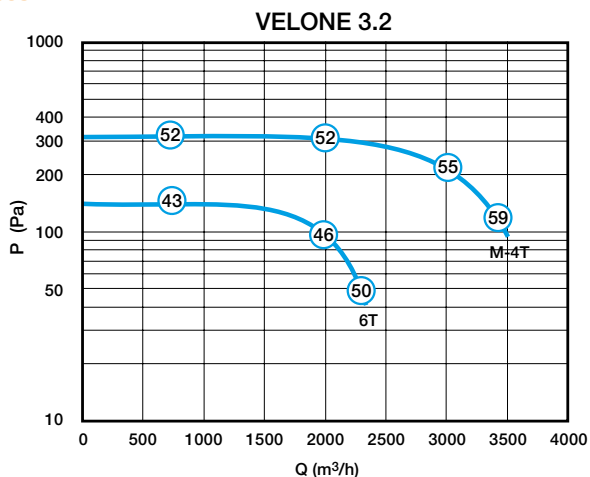
Caractéristiques aérauliques et acoustiques VELONE 3.2 - 4T 0.55 KW
