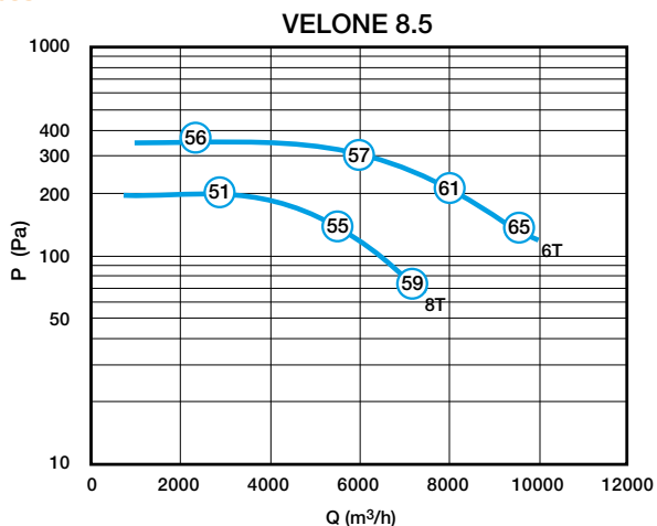
Caractéristiques aérauliques et acoustiques VELONE 8.5 - 6/12T 1.1/0.22 KW
