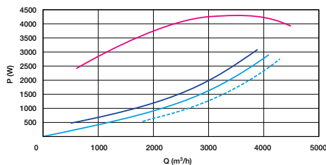
Débit et puissance VEX560-C4
